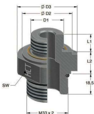
FORM 3 Abdichtung USIT-Ring
