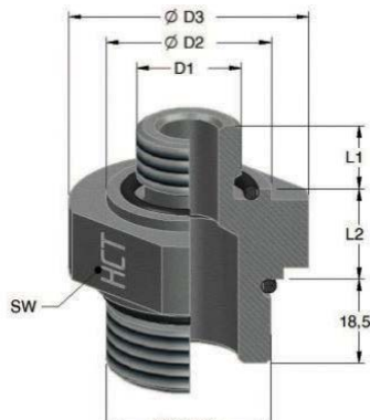
FORM 4 Abdichtung O-Ring
