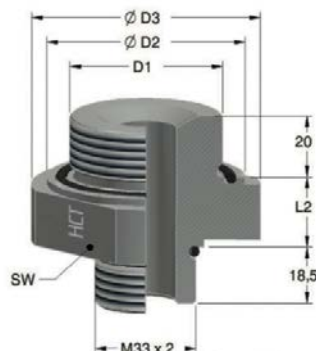
FORM 2 axiale Abdichtung
