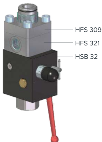
FORM 3 Zwischenflansch für zusätzl. seitlichen Rohranschluss
