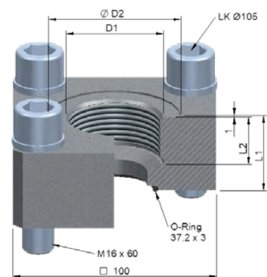
FORM 4 Flansch für Rohrleitungsanschluss
