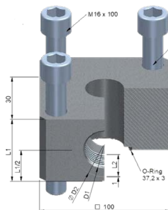
FORM 3 Zwischenflansch für zusätzl. seitlichen Rohranschluss
