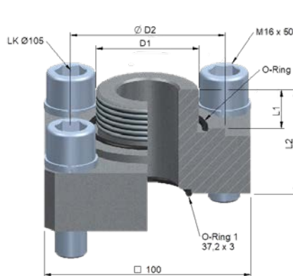
FORM 2 axiale Abdichtung
